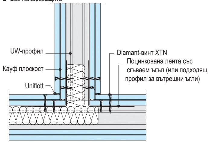
W112.bg-C2 T-връзки с гъвкав профил за ъгли/вътрешни ъгли
