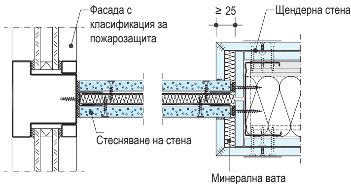
Стесняване на стена с пожарозащита - Вариант 3
