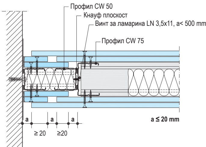
Стесняване на стена с пожарозащита - Вариант 3
