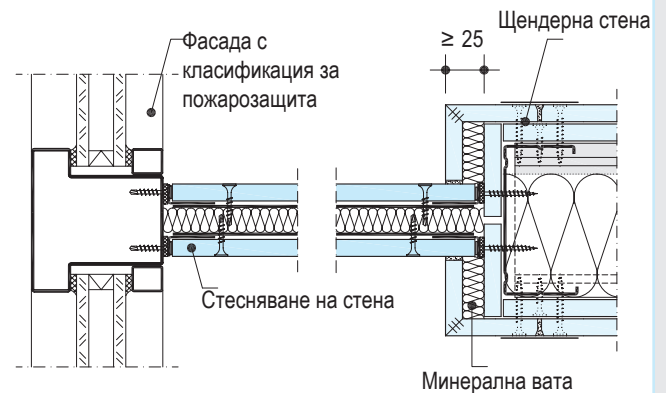
Стесняване на стена с пожарозащита - Вариант 6
