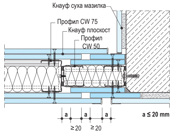
Стесняване на стена с пожарозащита - Вариант 6
